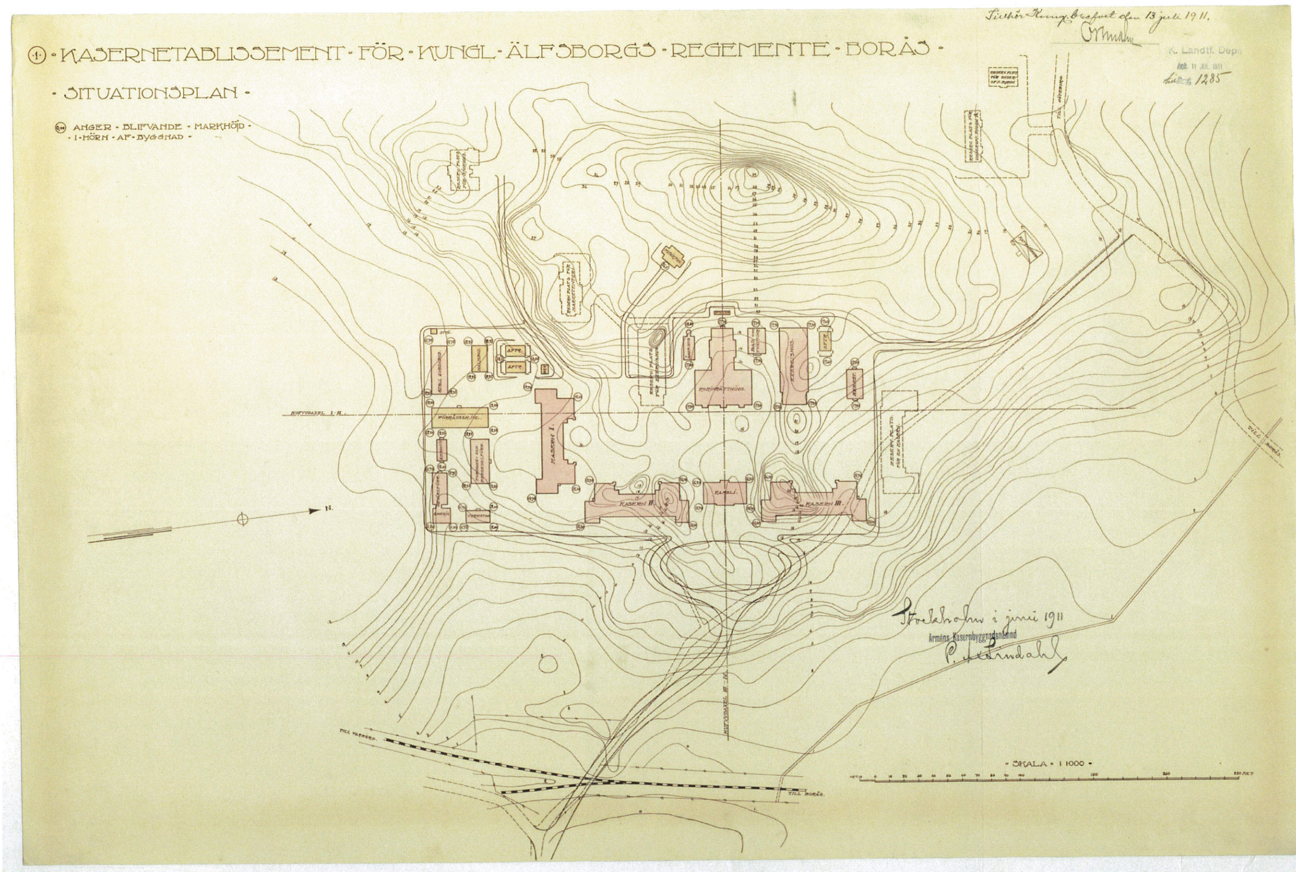
1, Ritning över planerat Kasernområde, f.d. Älvsborgs regemente, från 1911.
